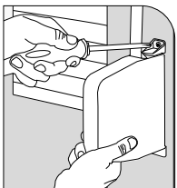
Mechanischen Gurtantrieb entfernen
